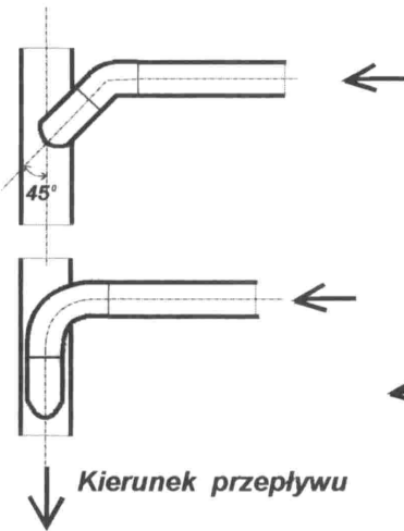
WIDOK W PLANIE
