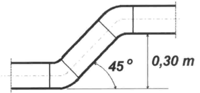
USKOK W PROFILU Dz 90 - 200 mm
