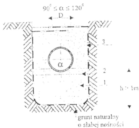
Rys. 4 Podłoże wzmocnione - grunty o głębokości zalegania powyżej 1 m
