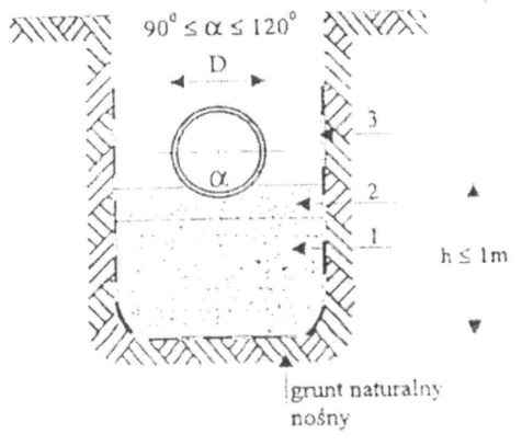
Rys. 3 Podłoże wzmocnione - grunty o głębokości zalegania do 1 m
