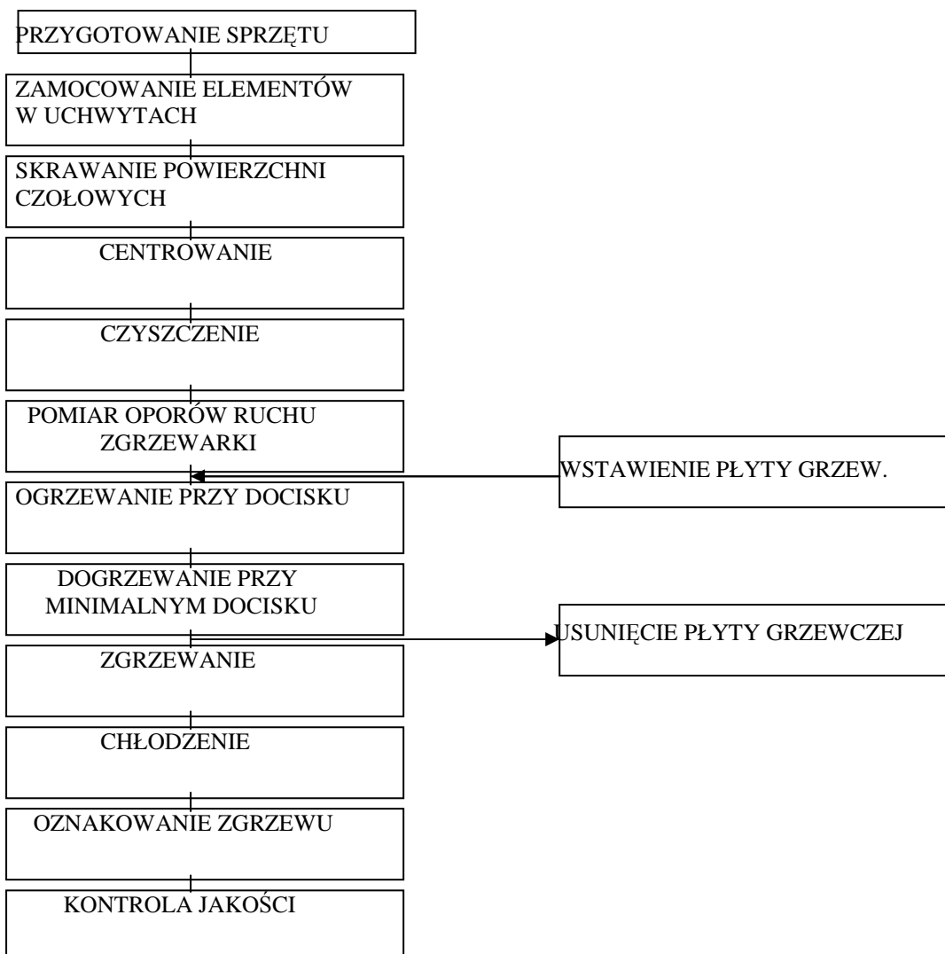
Rys. 1 Schemat blokowy zgrzewania czołowego
