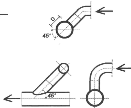
WIDOK W PROFILU
