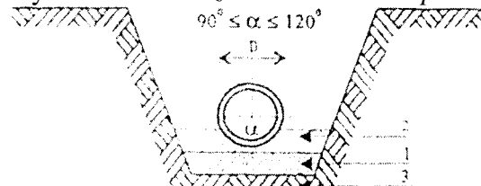
Rys. 2 Podłoże wzmocnione - ława piaskowa
