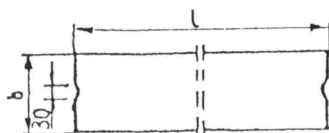
Rys. 1. Wymiarowanie krawężników
