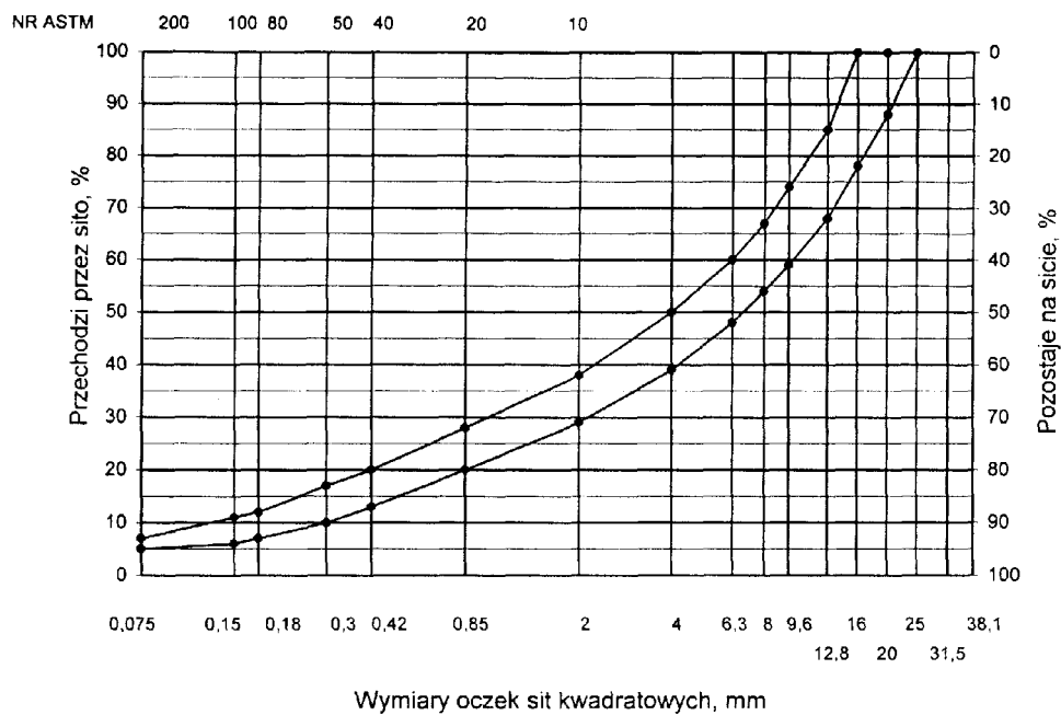
Wymiary oczek sit kwadratowych, mm Rys. 4. Krzywe graniczne uziarnienia mieszanki mineralnej BA od 0 do 20 mm do warstwy ścieralnej nawierzchni drogi o obciążeniu ruchem od KR3 do KR6
