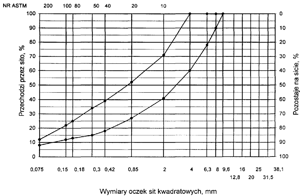
Wymiary oczek sit kwadratowych, mm Rys. 3. Krzywe graniczne uziarnienia mieszanki mineralnej BA od 0 do 8mm, od 0 do 6,3 mm do warstwy ścieralnej nawierzchni drogi o obciążeniu ruchem nawierzchni drogi o obciążeniu ruchem KR1 lub KR2
